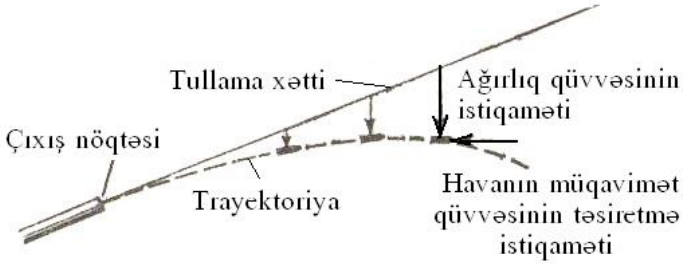
Güllənin uçuş trayektoriyası (yan tərəfdən görünüşü).
