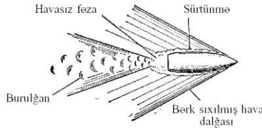
Havanın müqavimət qüvvəsinin əmələ gəlməsi.
